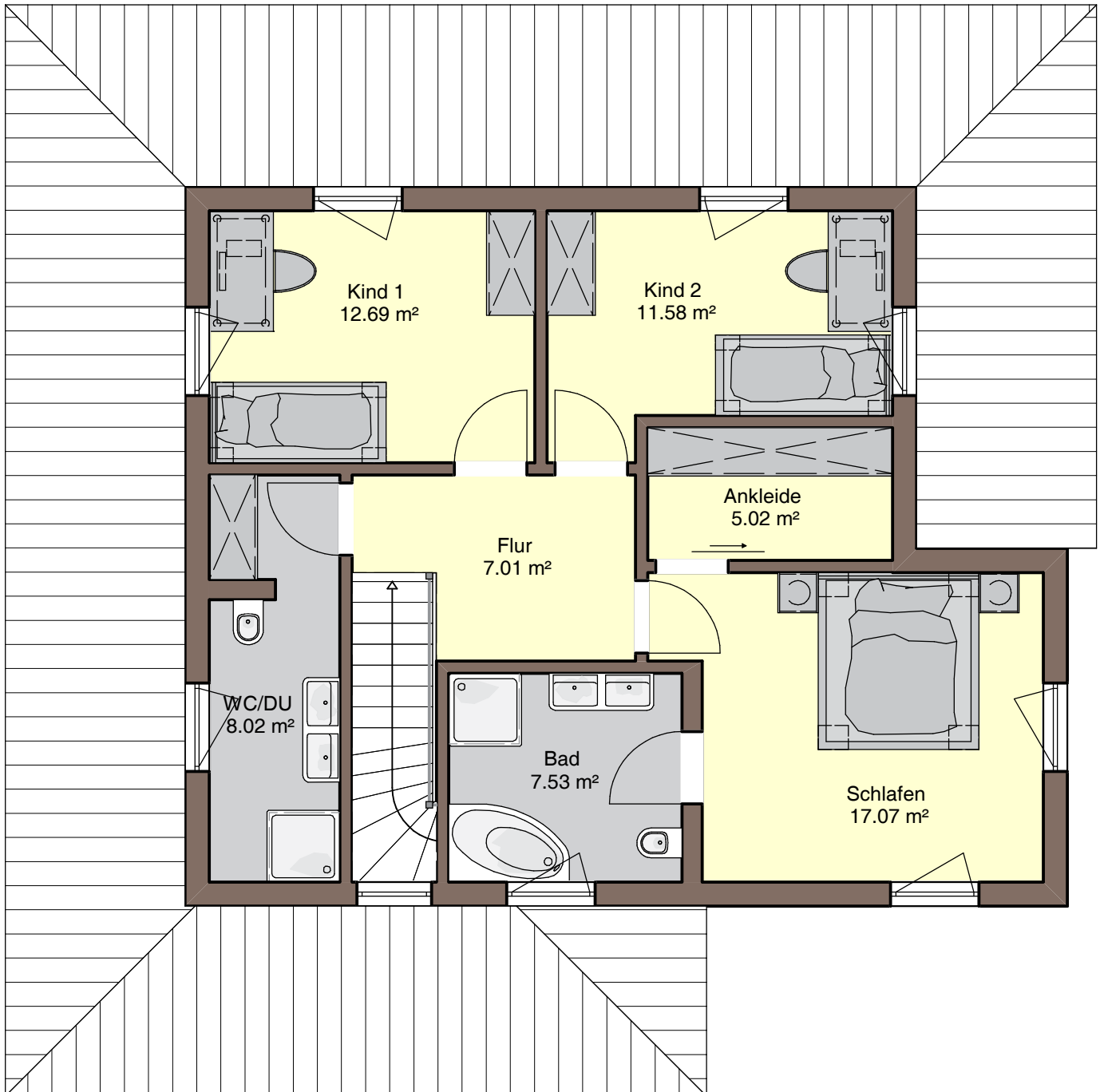
Dachgeschoss
