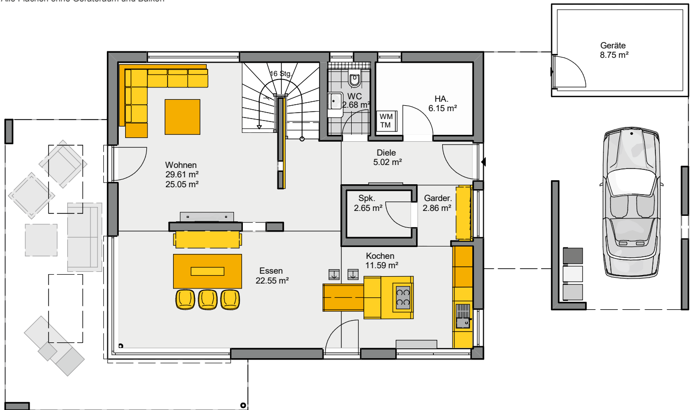
Erdgeschoss
