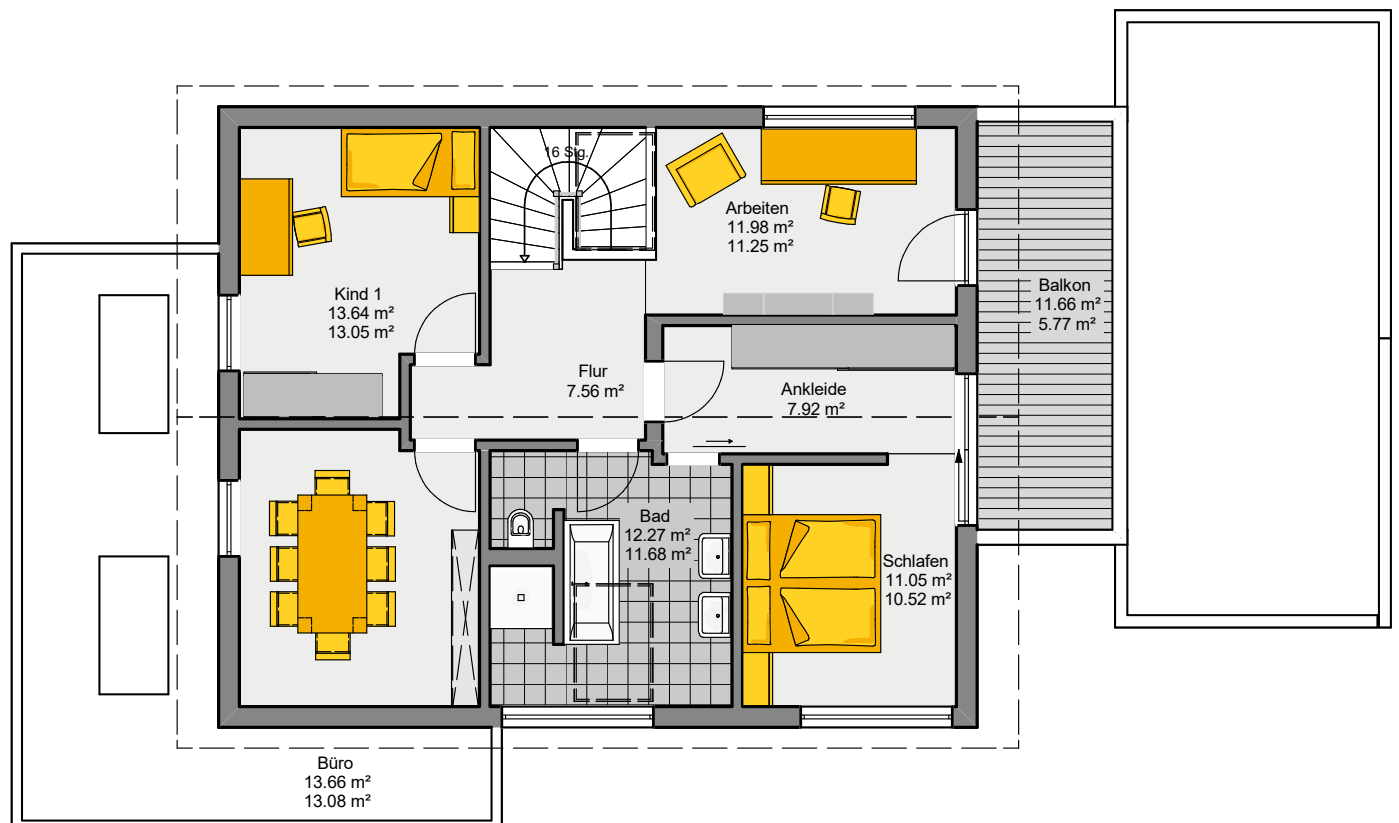
Dachgeschoss
